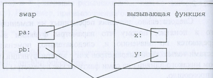
Рис. 3. Работа функции swap
