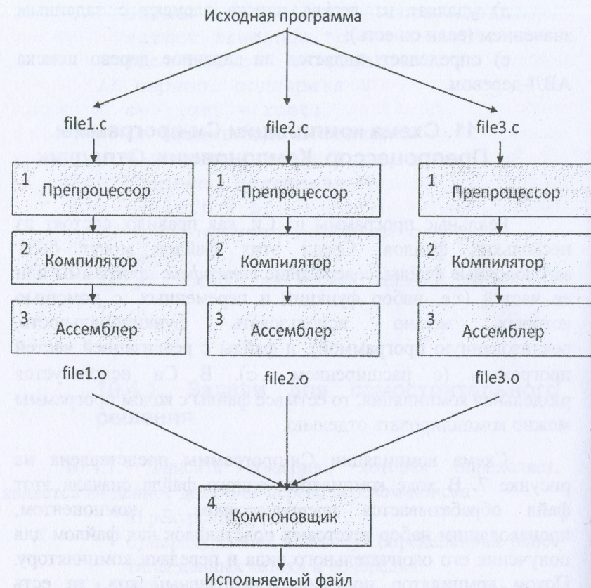
Рис. 7. Схема компиляции многомодульной программы.
