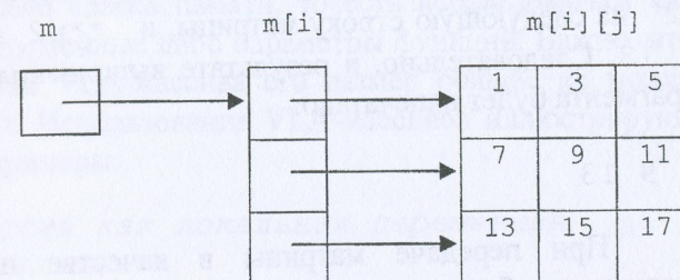
Рис. 4. Доступ к элементам матрицы
