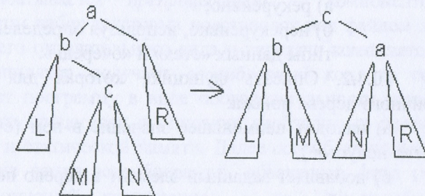
Рис. 6. Балансировка AVL-дерева
